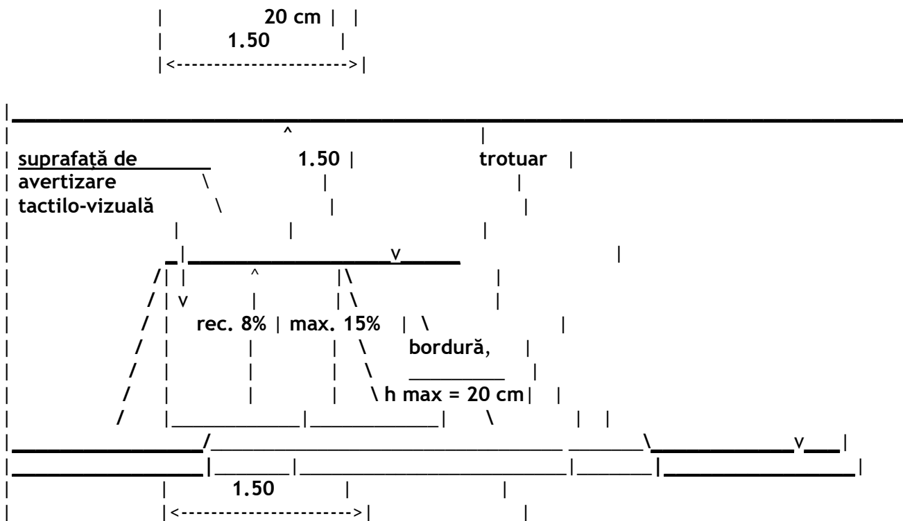
Fig. IV.8. - Rampă de acces între trotuar și carosabil
