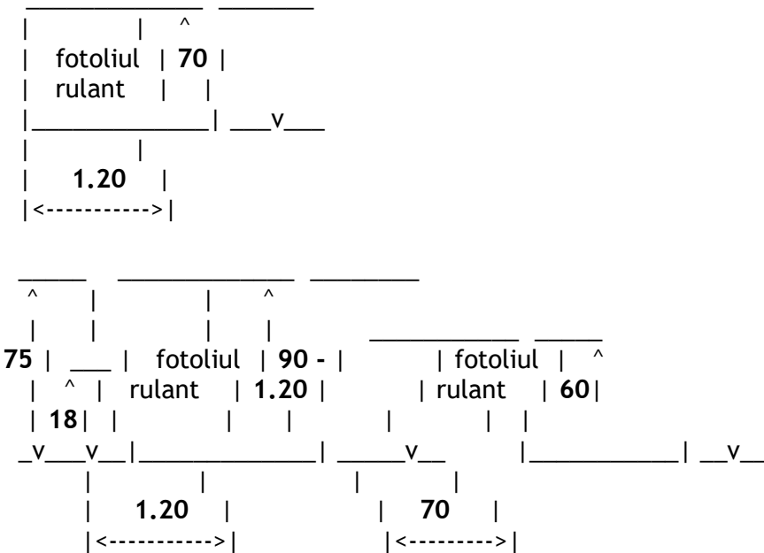
Fig. III.3. - Dimensiuni ale fotoliului rulant - persoane adulte
