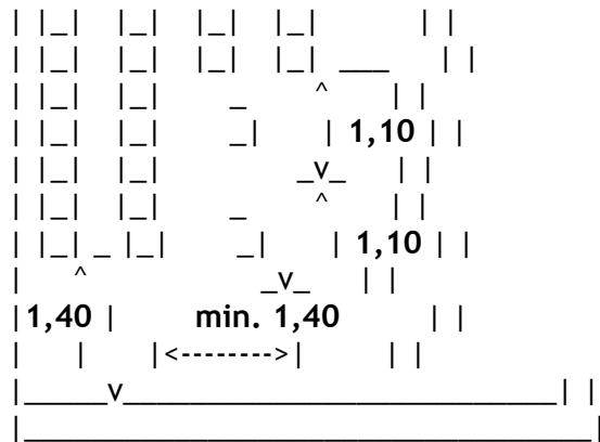
Fig. VII.1. a. - Amplasarea în cadrul unei săli de spectacole a locurilor rezervate persoanelor cu handicap
